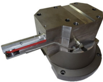
Schleifkopf mit Drehzahlübersetzung
